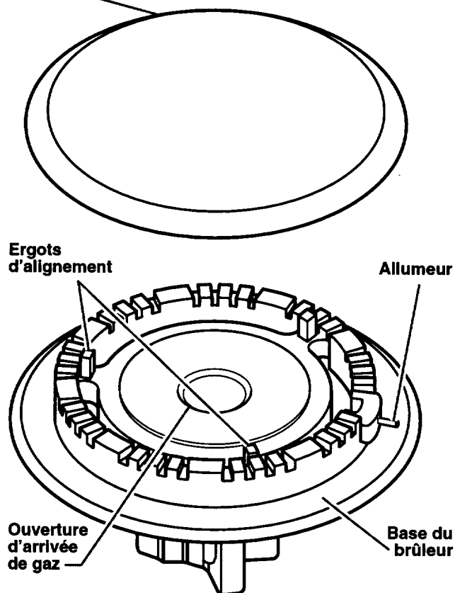
Chapeau de brûleur, en fonte
